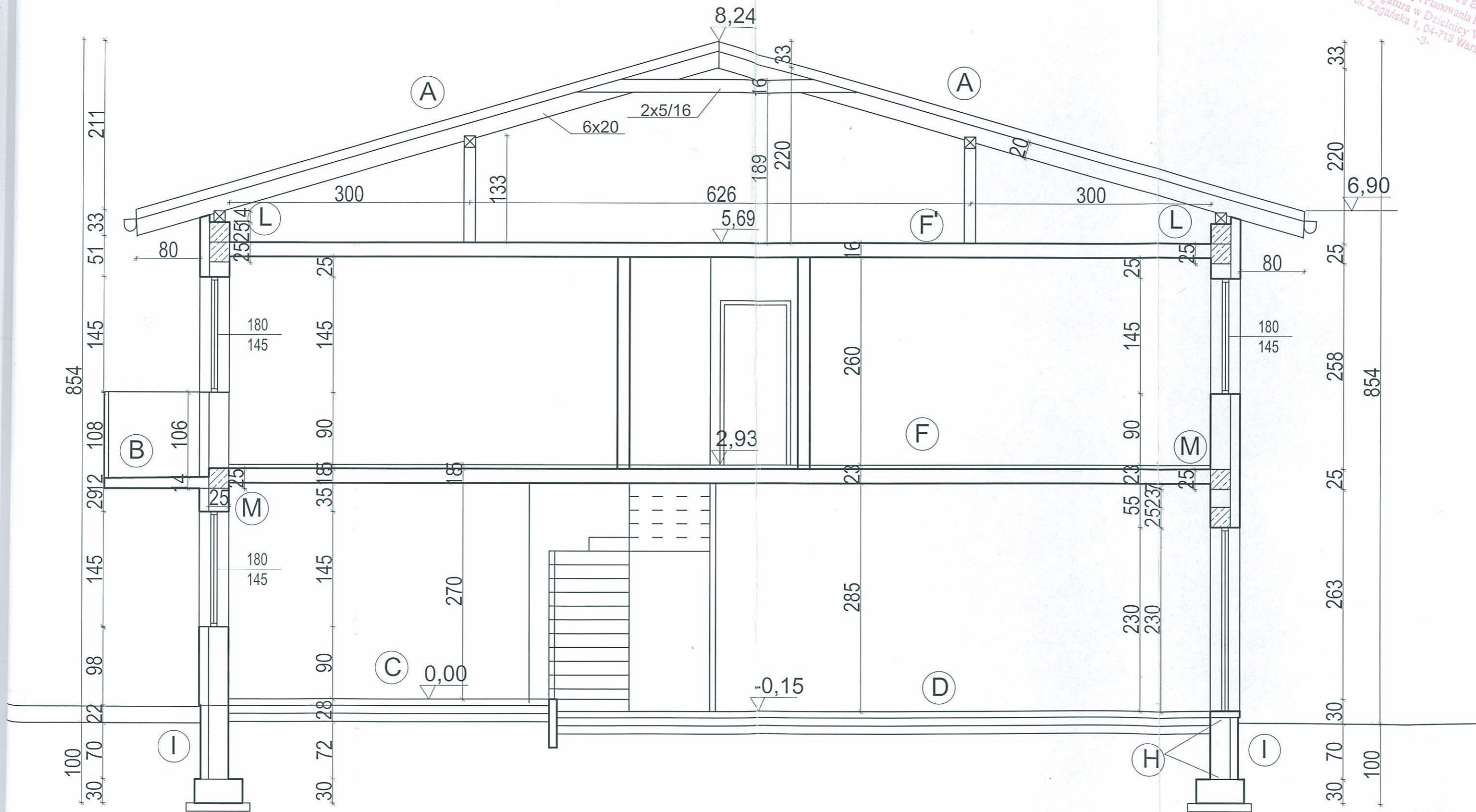
PRZEKRÓJ A-A
